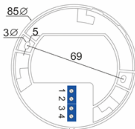
Рисунок 130. Установочный чертеж RF05-ДО, RF05-ДО/И, RF05-Т
