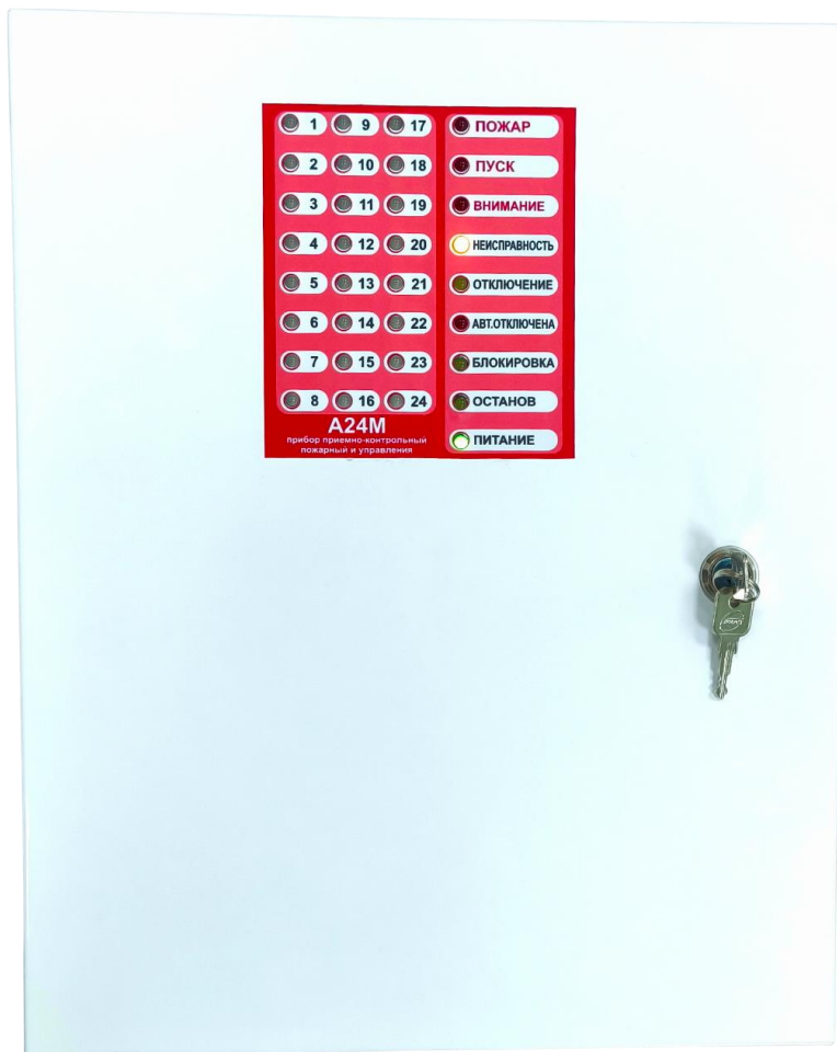
Рисунок 4. Внешний вид ППКПиУ исполнения «А24М» с закрытой лицевой панелью
