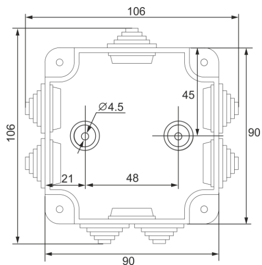
Рисунок 124. Установочный чертеж БУН1-12С
