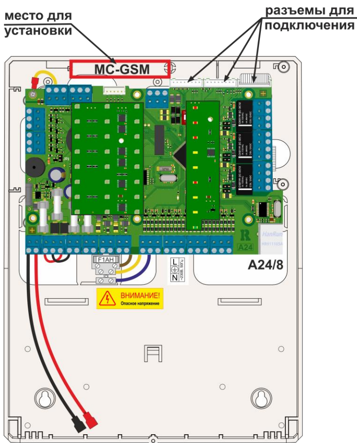
Рисунок 108. Установка и подключение MC-GSM к ППКПиУ исполнений «A24» и «A24E»
