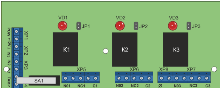
Рисунок 104. Внешний вид платы и обозначение элементов БУН3-12
