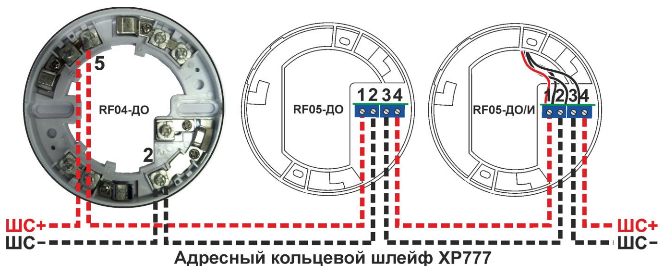
Рисунок 112. Схема подключения RF04-ДО, RF05-ДО, RF05-ДО/И
