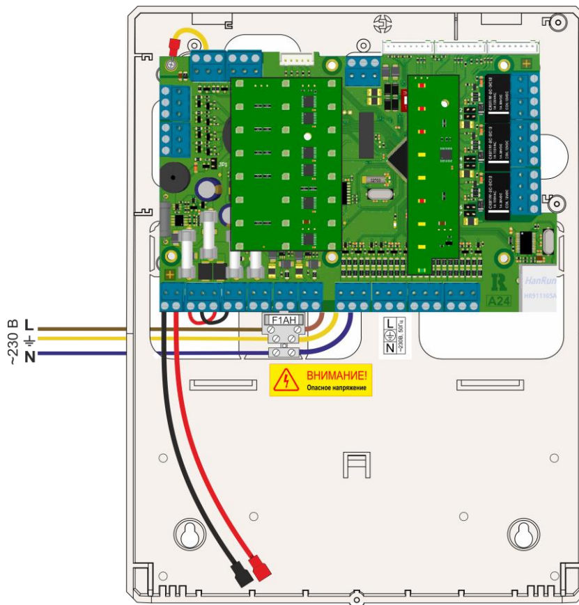
Рисунок 8. Схема подключения основного питания к ППКПиУ исполнений «A24» и «A24E»
