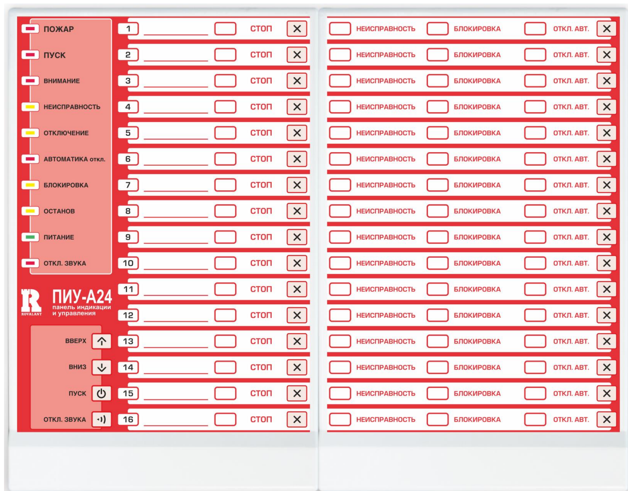
Рисунок 88. Внешний вид ПИУ-A24А
