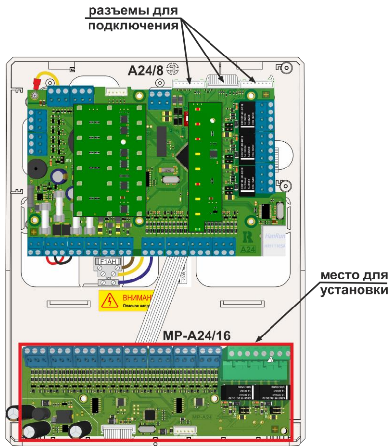
Рисунок 11. Установка и подключение MP-A24/16 к ППКПиУ исполнений «A24», «A24E»
