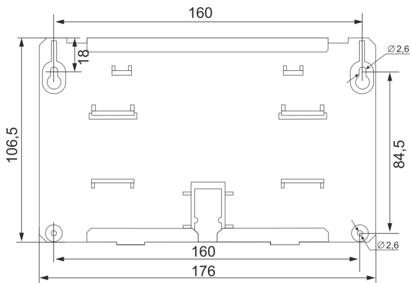
Рисунок 127. Установочный чертеж P485 и RS485/FTTx-S-SC
