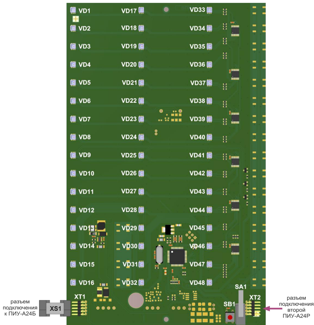
Рисунок 87. Внешний вид и подключение платы ПИУ-A24P
