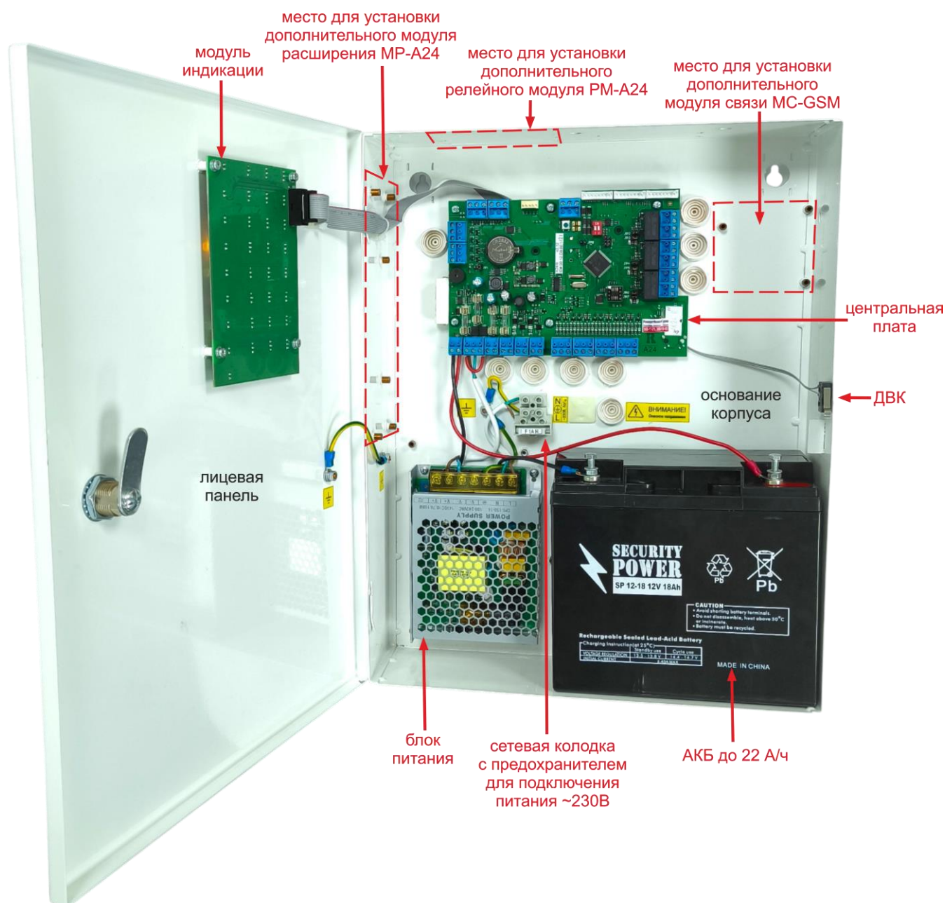
Рисунок 5. ППКПиУ «А24М» с открытой лицевой панелью
