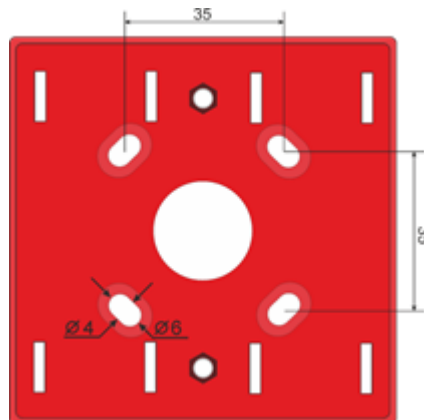
Рисунок 131. Установочный чертеж RF04-P
