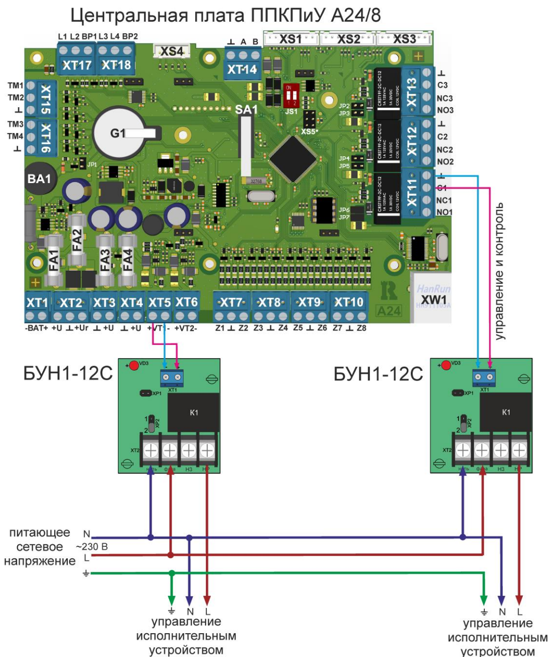
Рисунок 100. Схема подключения БУН1-12С к ППКПиУ А24/8.
