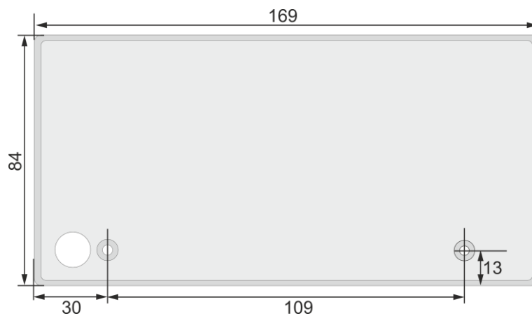
Рисунок 128. Установочный чертеж БУНЗ-12
