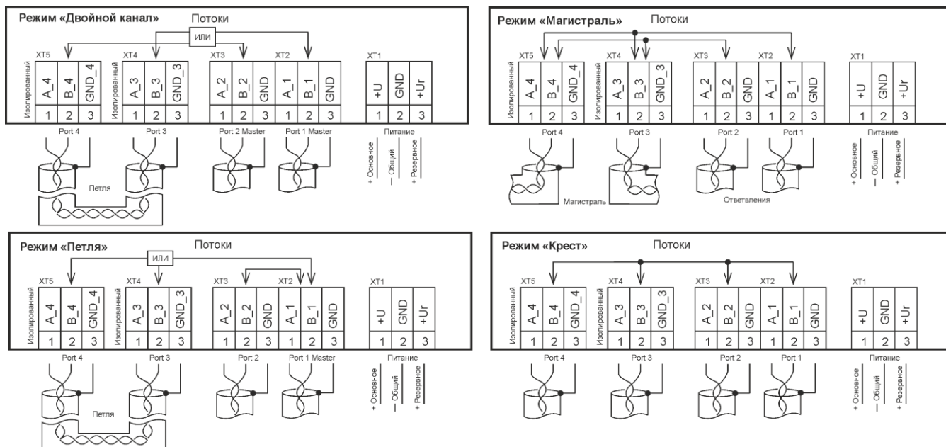
Рисунок 92. Подключение P485 при различных режимах его работы
