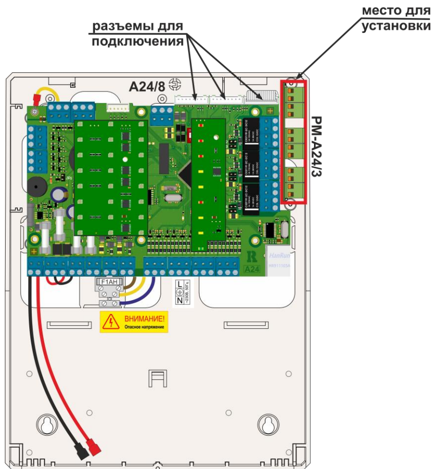
Рисунок 16. Установка и подключение PM-A24/3 к ППКПиУ исполнений «A24», «A24E»
