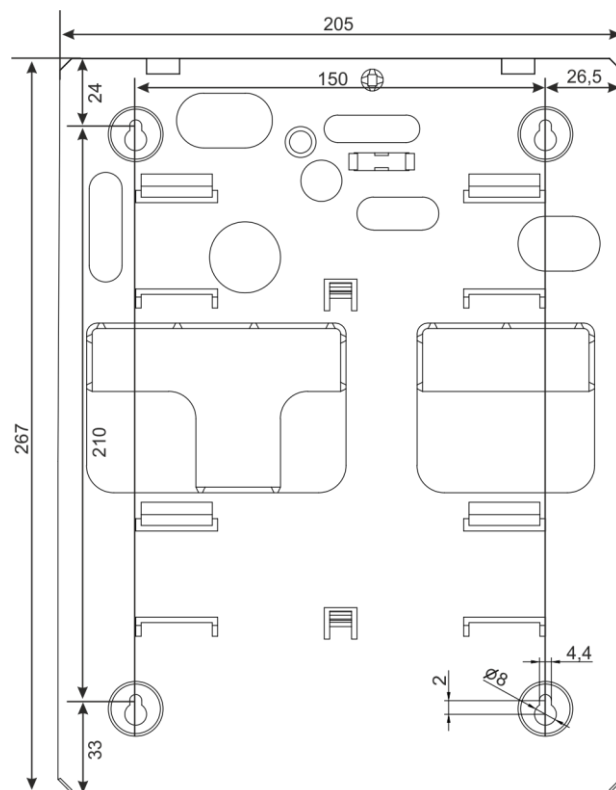
Рисунок 120. Установочный чертеж ППКПиУ исполнений «А24», «А24Е» и БА-18
