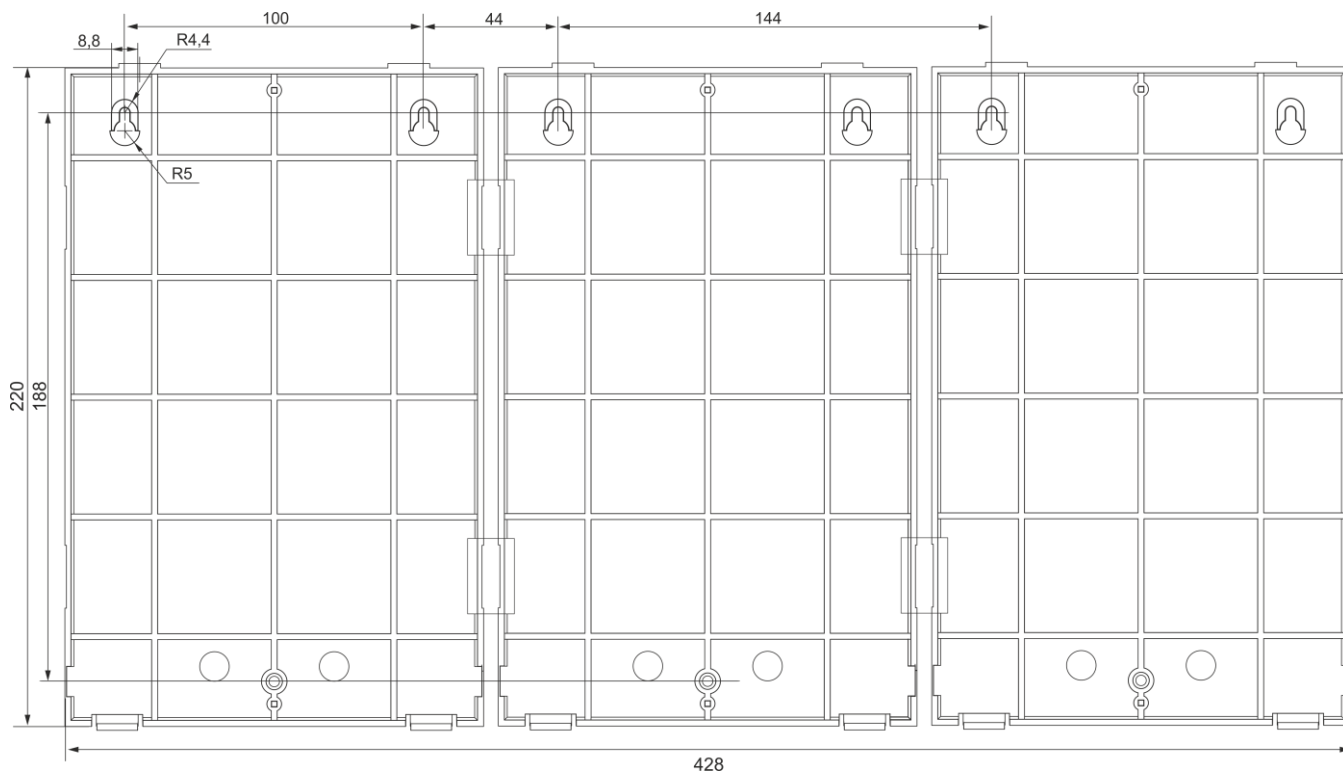
Рисунок 126. Установочный чертеж ПИУ-A24Б при применении с двумя ПИУ-A24Р
