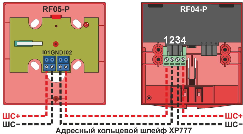
Рисунок 119. Схема подключения RF04-P, RF05-P
