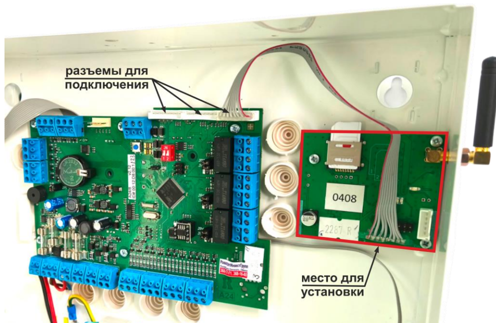
Рисунок 109. Установка MC-GSM в корпус ППКПиУ исполнения «А24М»
