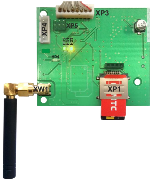
Рисунок 110. Внешний вид и обозначение элементов MC-GSM
