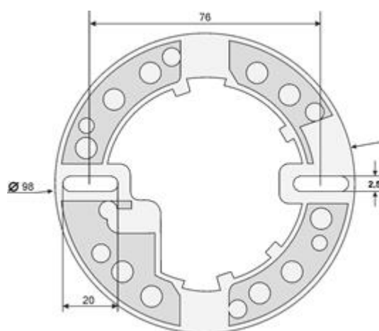
Рисунок 129. Установочный чертеж RF04-ДО, ИП101-02-ВМ, изолирующего основания XR777
