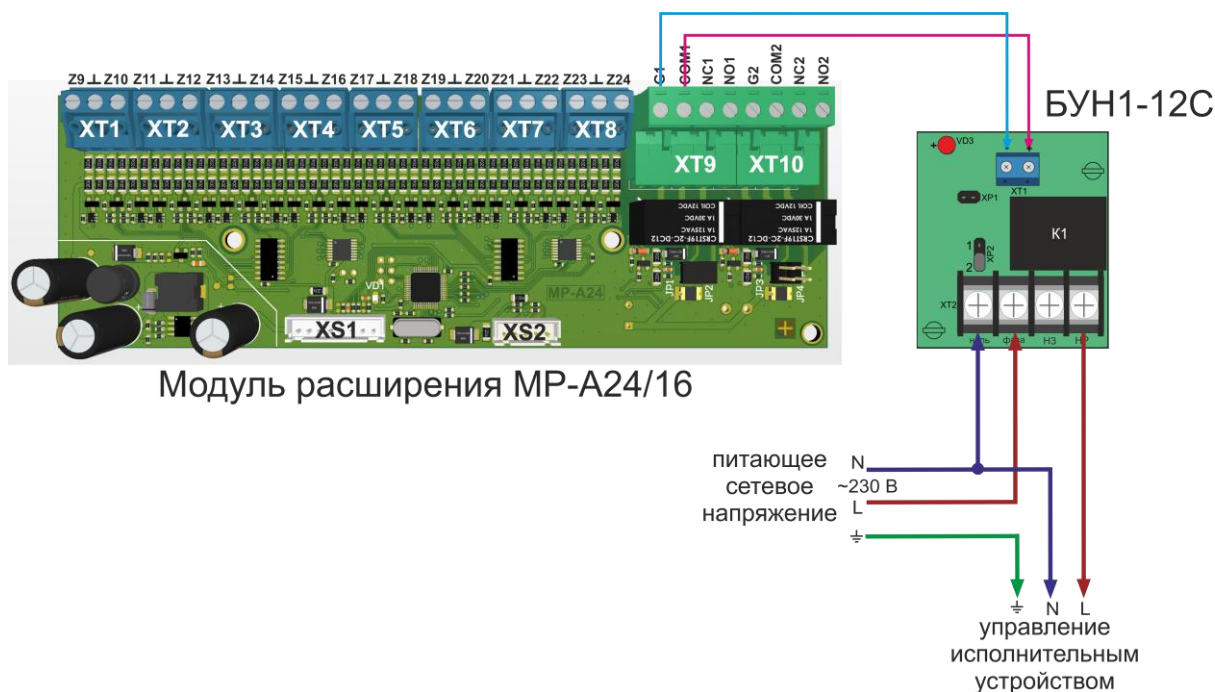
Рисунок 101. Схема подключения БУН1-12С к MP-A24/16.
