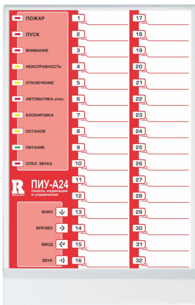
Рисунок 83. Внешний вид ПИУ-А24Б
