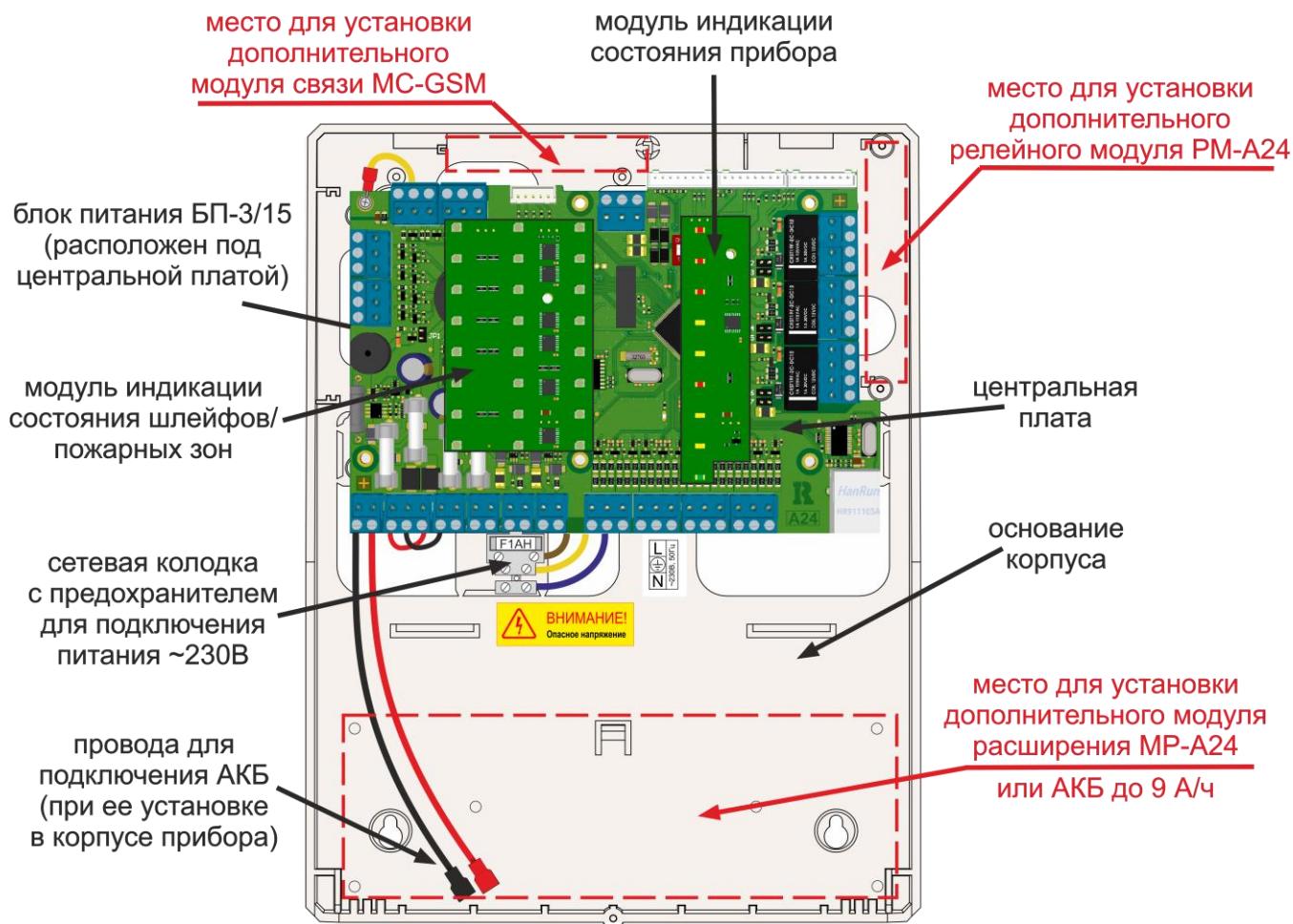
Рисунок 3. ППКПиУ исполнений «А24» и «А24Е» с открытой передней крышкой
