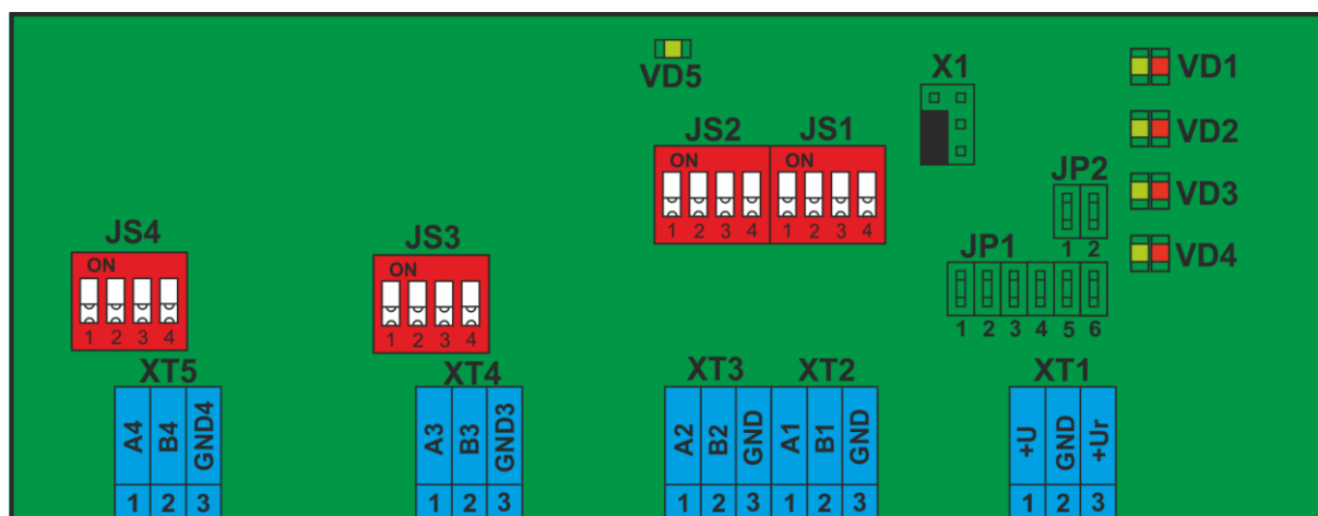
Рисунок 91. Внешний вид платы Р485
