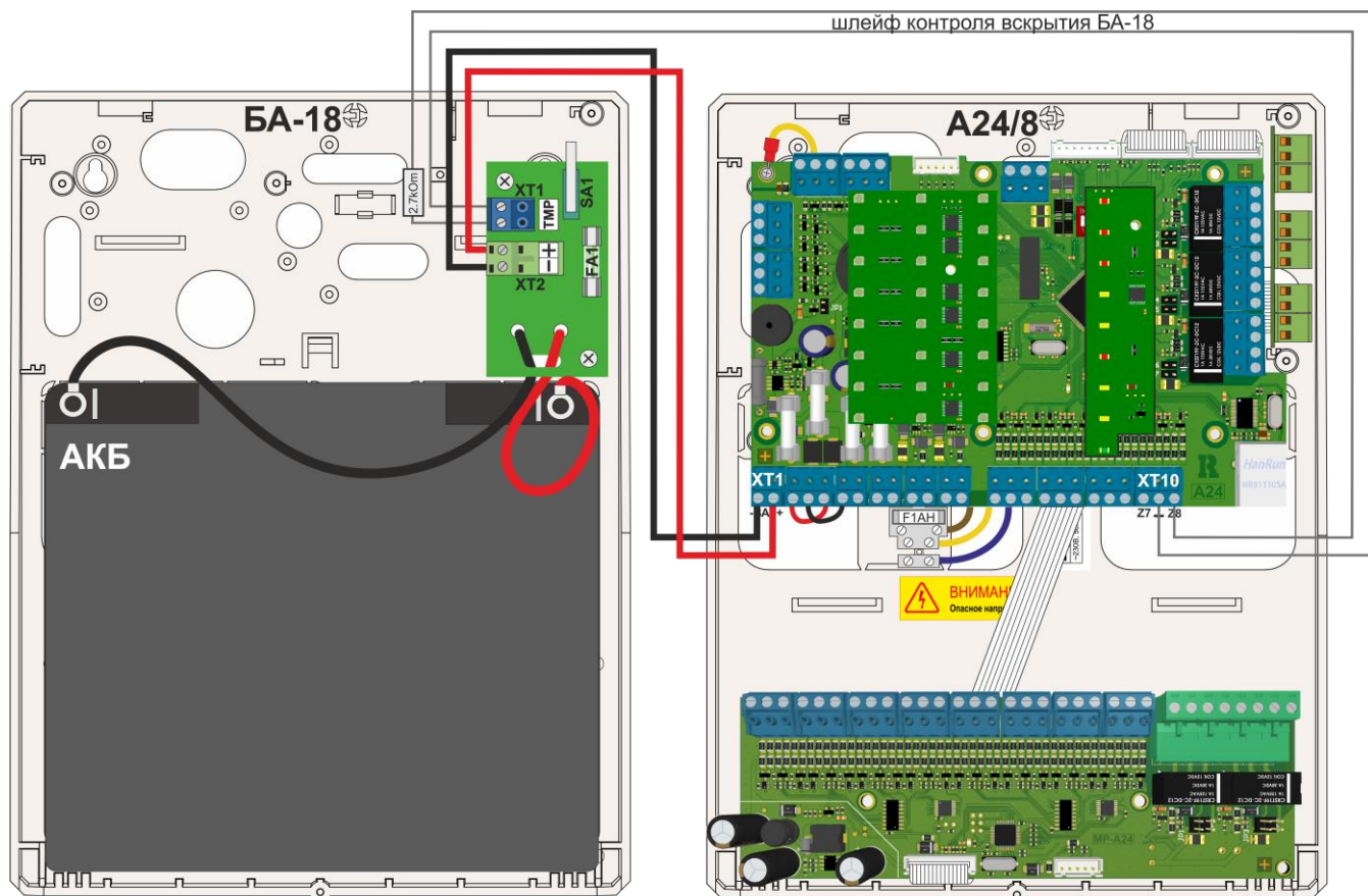
Рисунок 107. Схема подключения БА-18 к ППКПиУ А24/8.
