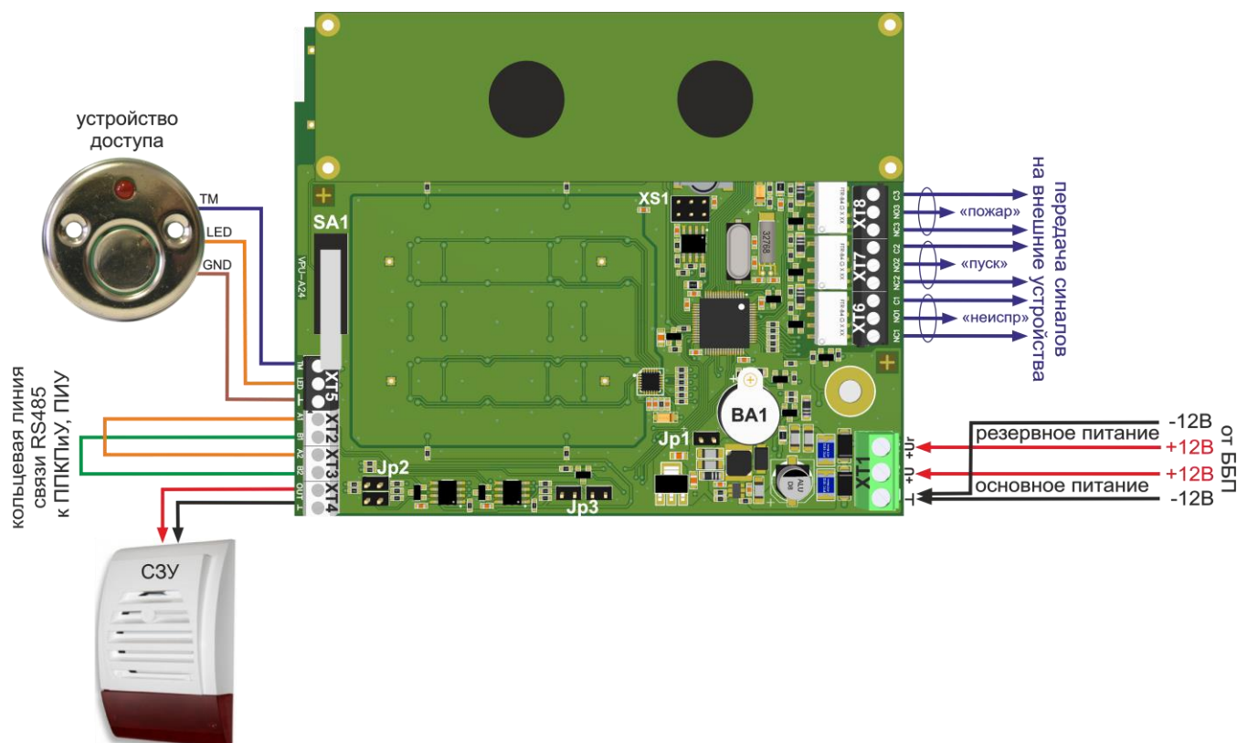
Рисунок 21. Схема подключения ВПУ-А24/700
