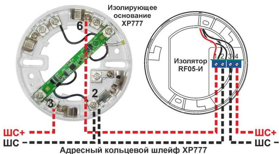
Рисунок 117. Схема подключения изолирующего основания XR777 и изолятора коротких замыканий RF05-И.
