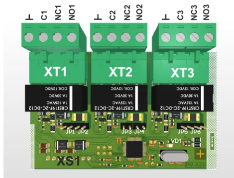
Рисунок 15. Внешний вид и обозначение элементов РМ-А24/3
