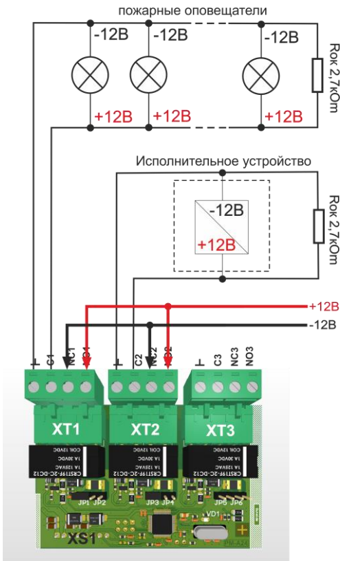
Рисунок 18. Схема подключения РМ-А24/3
