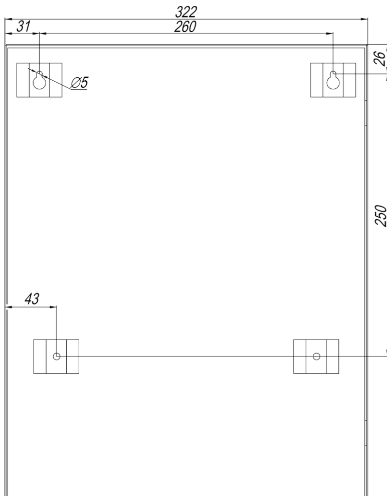
Рисунок 121. Установочный чертеж ППКПиУ исполнения «А24М»
