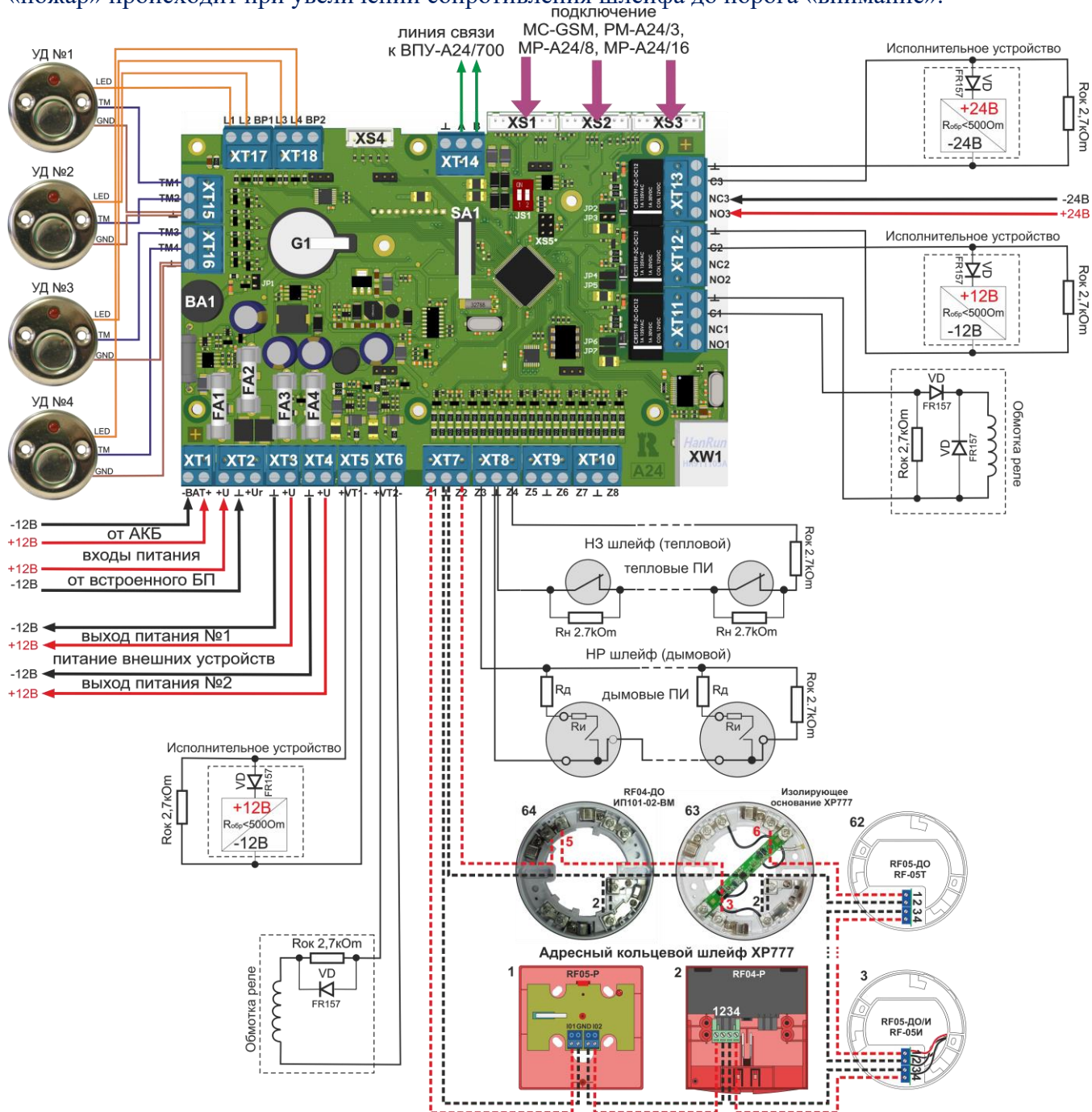
Рисунок 10. Пример схемы подключения A24/8
