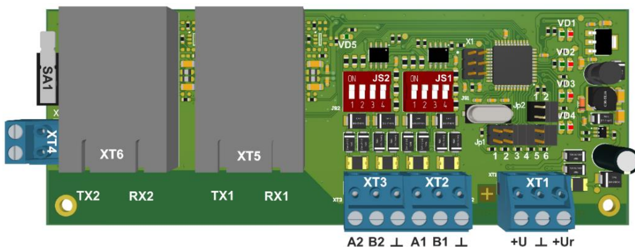
Рисунок 95. Внешний вид платы RS485/FTTx-S-SC
