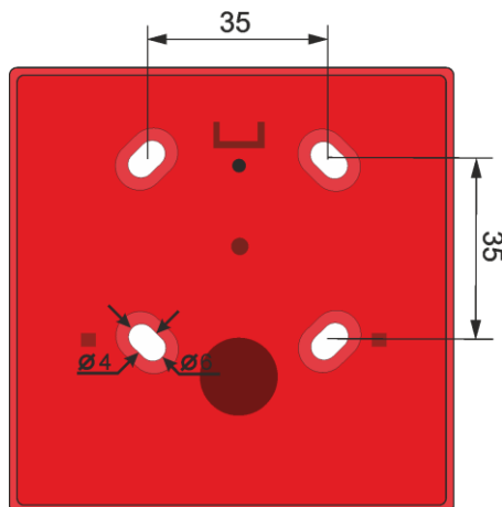
Рисунок 132. Установочный чертеж RF05-P
