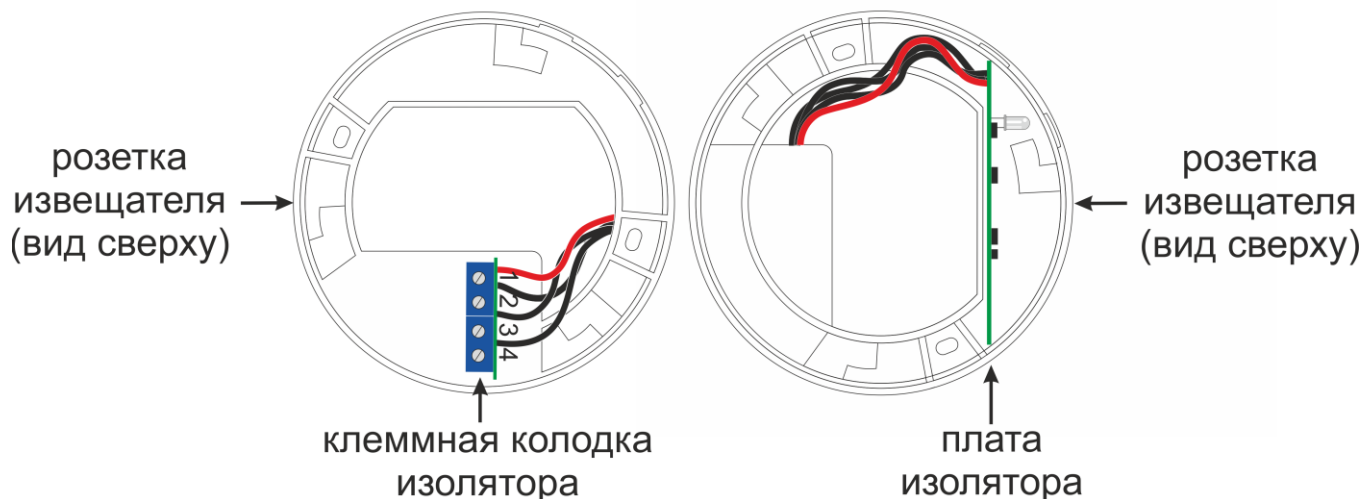
Рисунок 116. Установка RF05-И в розетку извещателя
