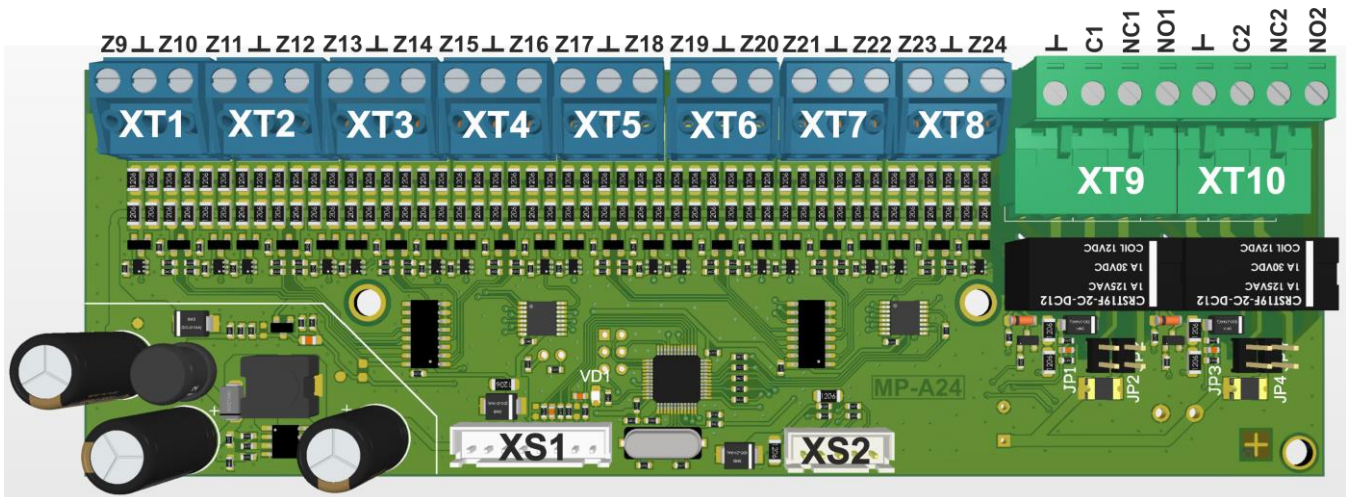
Рисунок 13. Внешний вид и обозначение элементов МР-А24/16
