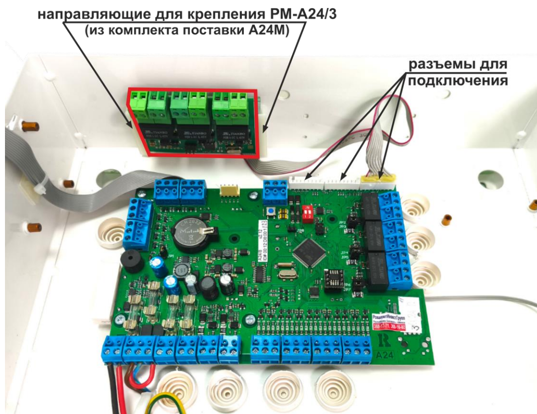
Рисунок 17. Установка и подключение PM-A24/3 к ППКПиУ исполнения «A24M»
