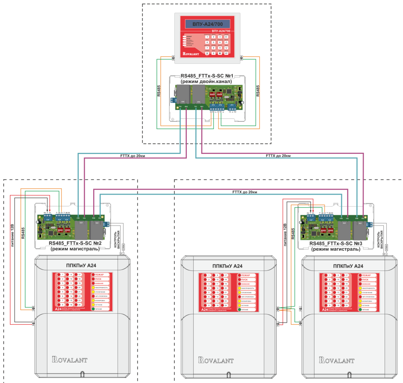
Рисунок 98. Схема организации оптоволоконной линии связи между ВПУ-A24/700 и приборами серии «A24»
