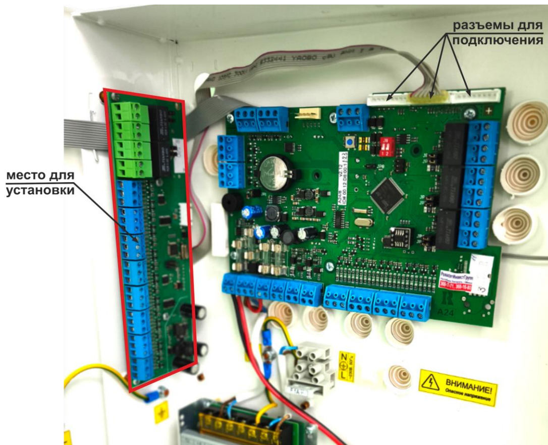
Рисунок 12. Установка и подключение MP-A24/16 к ППКПиУ исполнения «A24M»
