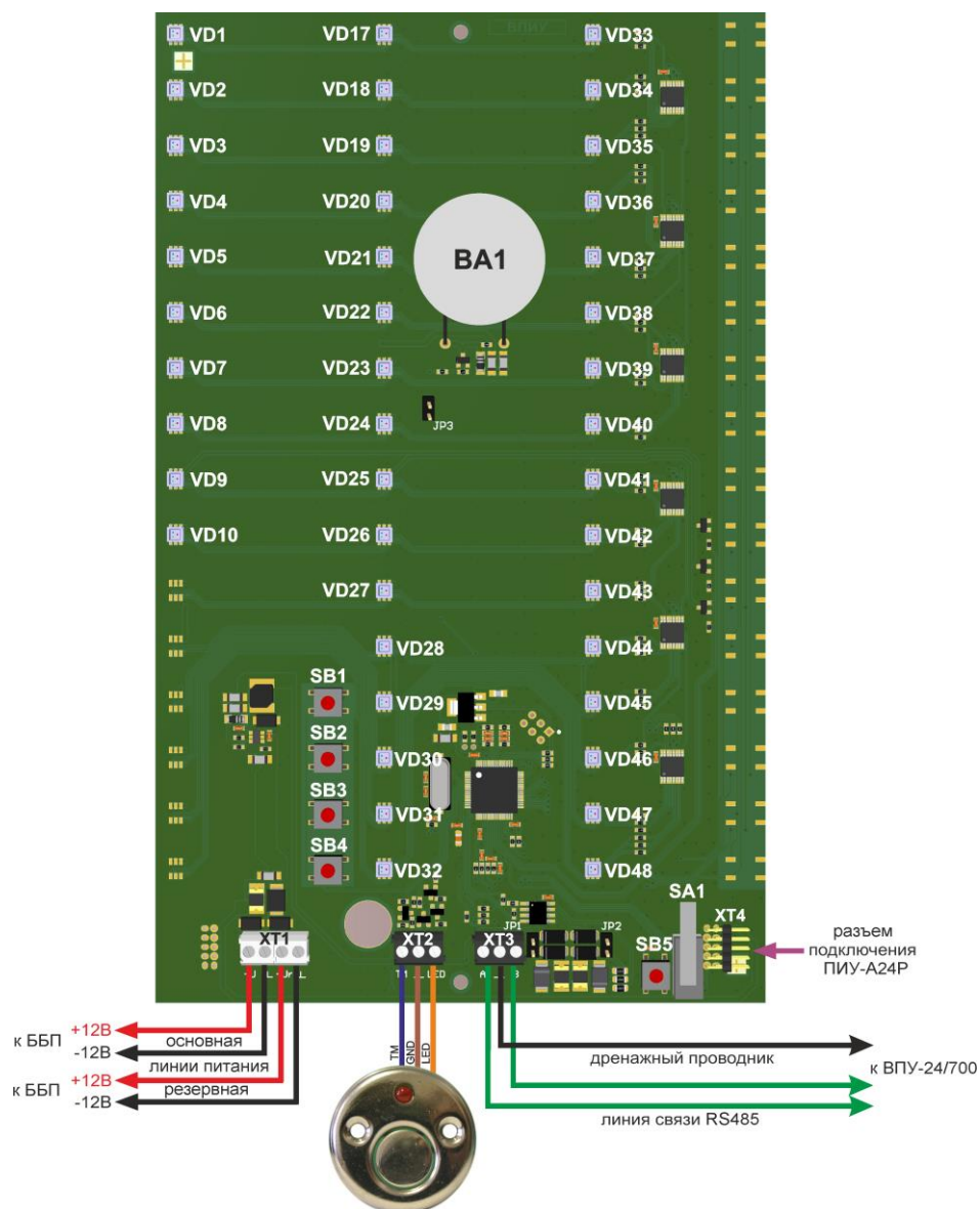
Рисунок 84. Внешний вид и подключение платы ПИУ-А24Б
