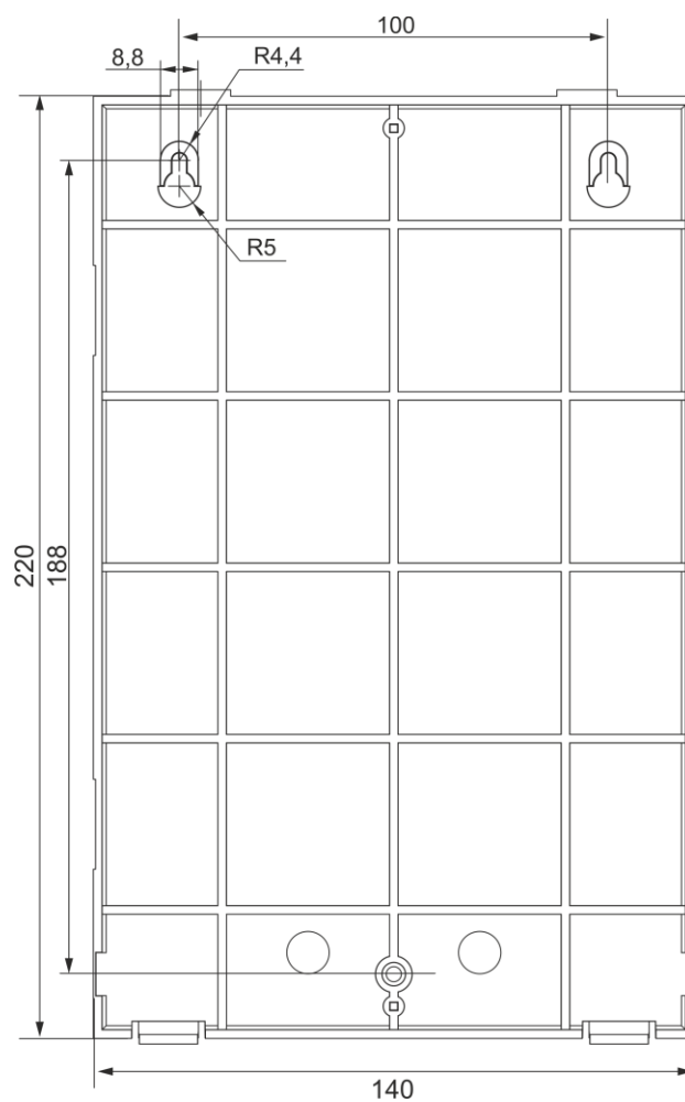
Рисунок 123. Установочный чертеж ПИУ-А24Б
