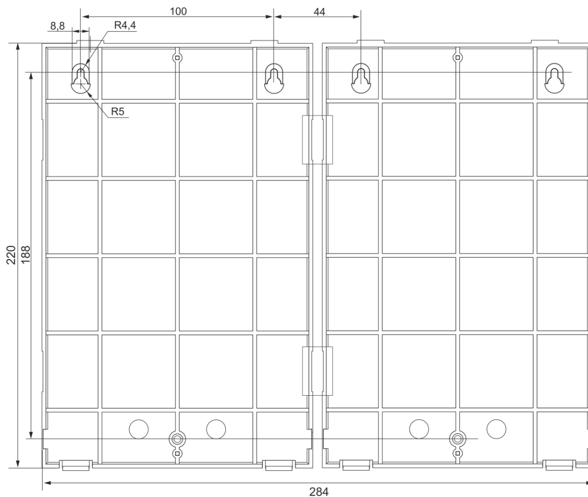
Рисунок 125. Установочный чертеж ПИУ-А24А или ПИУ-А24Б при применении совместно с одной ПИУ-А24Р
