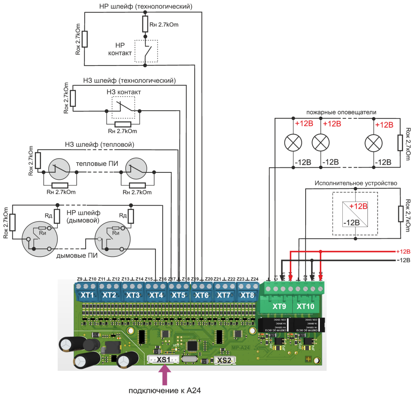
Рисунок 14. Схема подключения МР-А24/16
