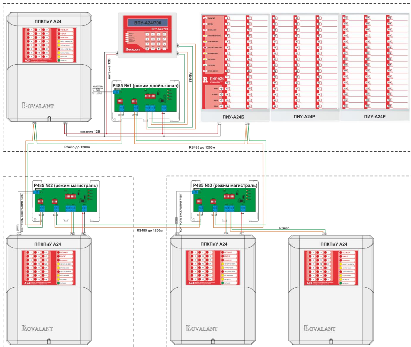
Рисунок 93. Схема подключения P485 для организации кольцевой гальвано-развязанной линии связи с сегментированной защитой от коротких замыканий.
