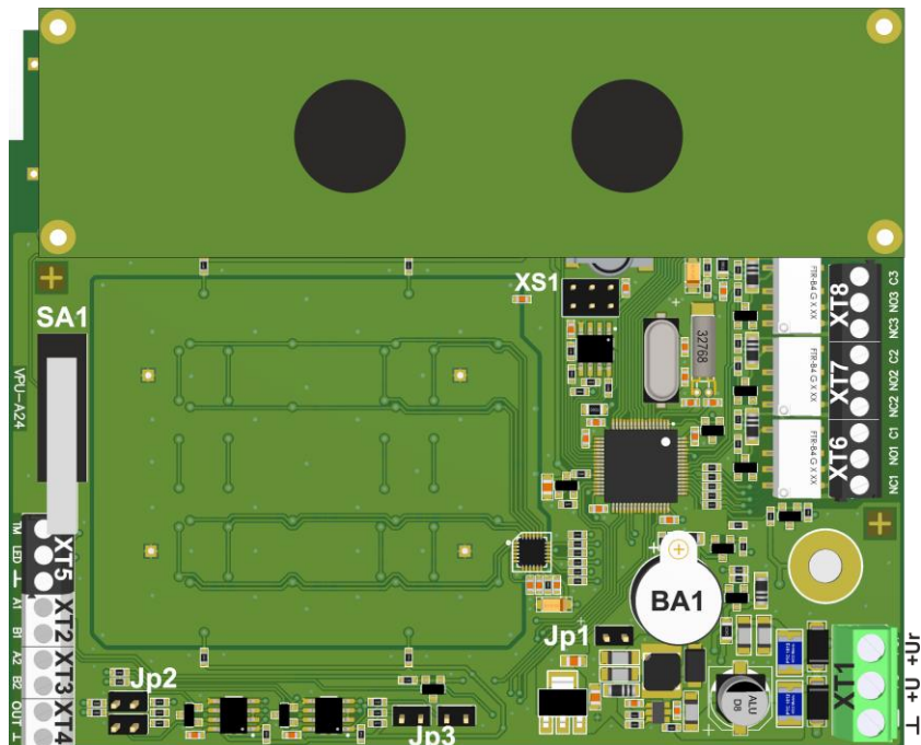
Рисунок 20. Внешний вид и обозначение элементов платы ВПУ-А24/700.
