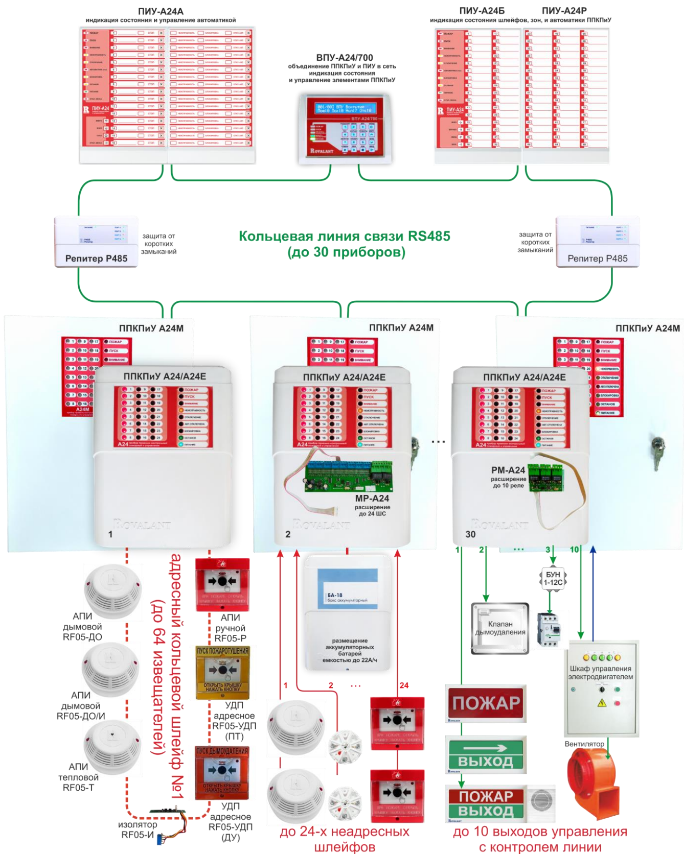
Рисунок 1. Структурная схема ПЖКПиУ и компонентов
