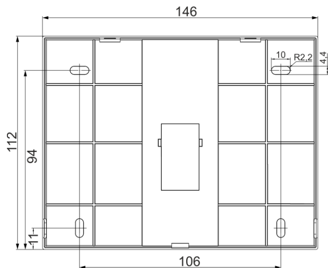
Рисунок 122. Установочный чертеж ВПУ-А24/700
