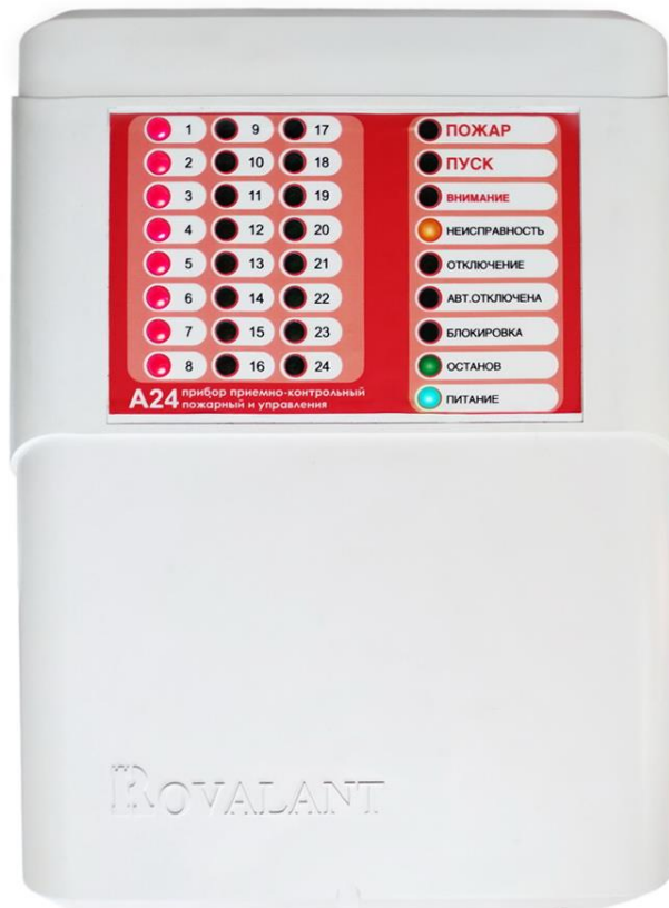
Рисунок 2. Внешний вид ППКПиУ исполнений «А24» и «А24Е» с закрытой передней крышкой
