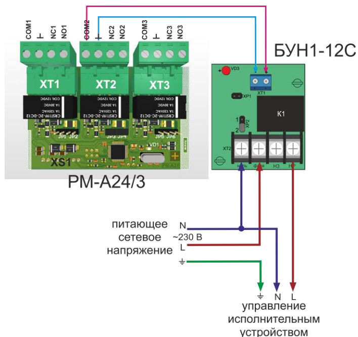
Рисунок 102. Схема подключения БУН1-12С к РМ-А24/3.
